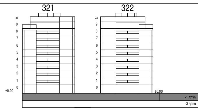
חותך סכמטי
