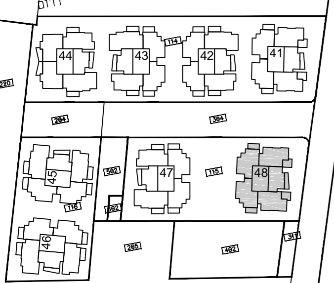
תכנית העמדה סכמטית מתחם ד
