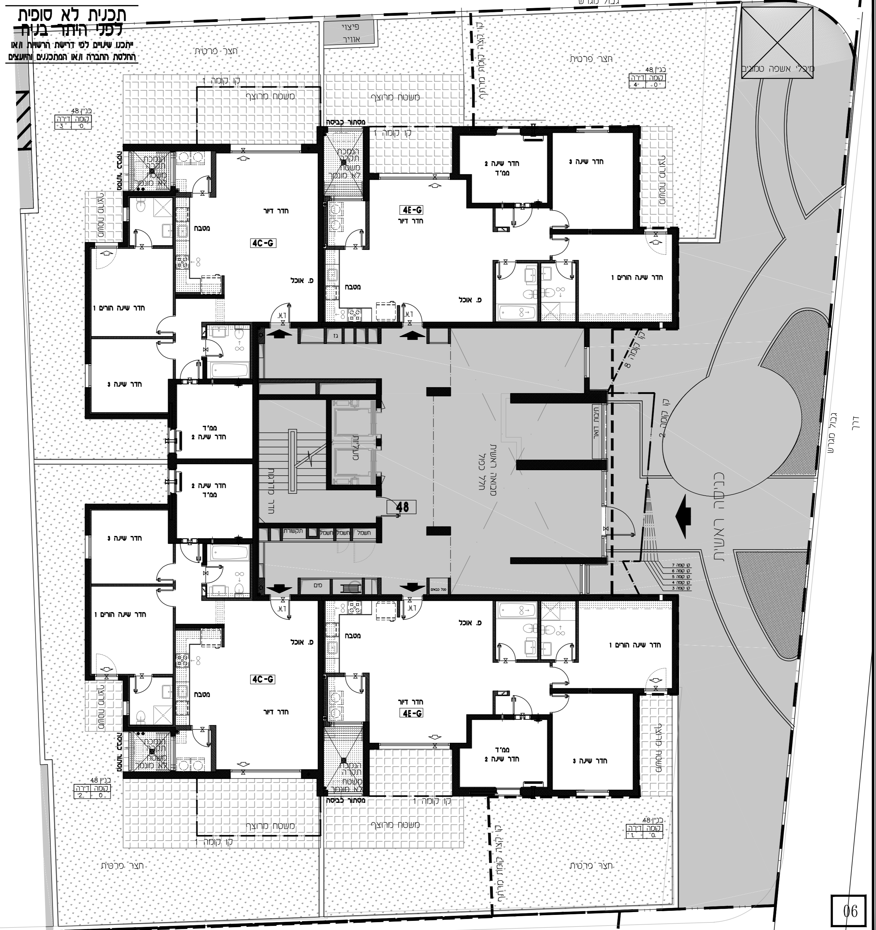
תכנית העמדה סכמטית מתחם ד
