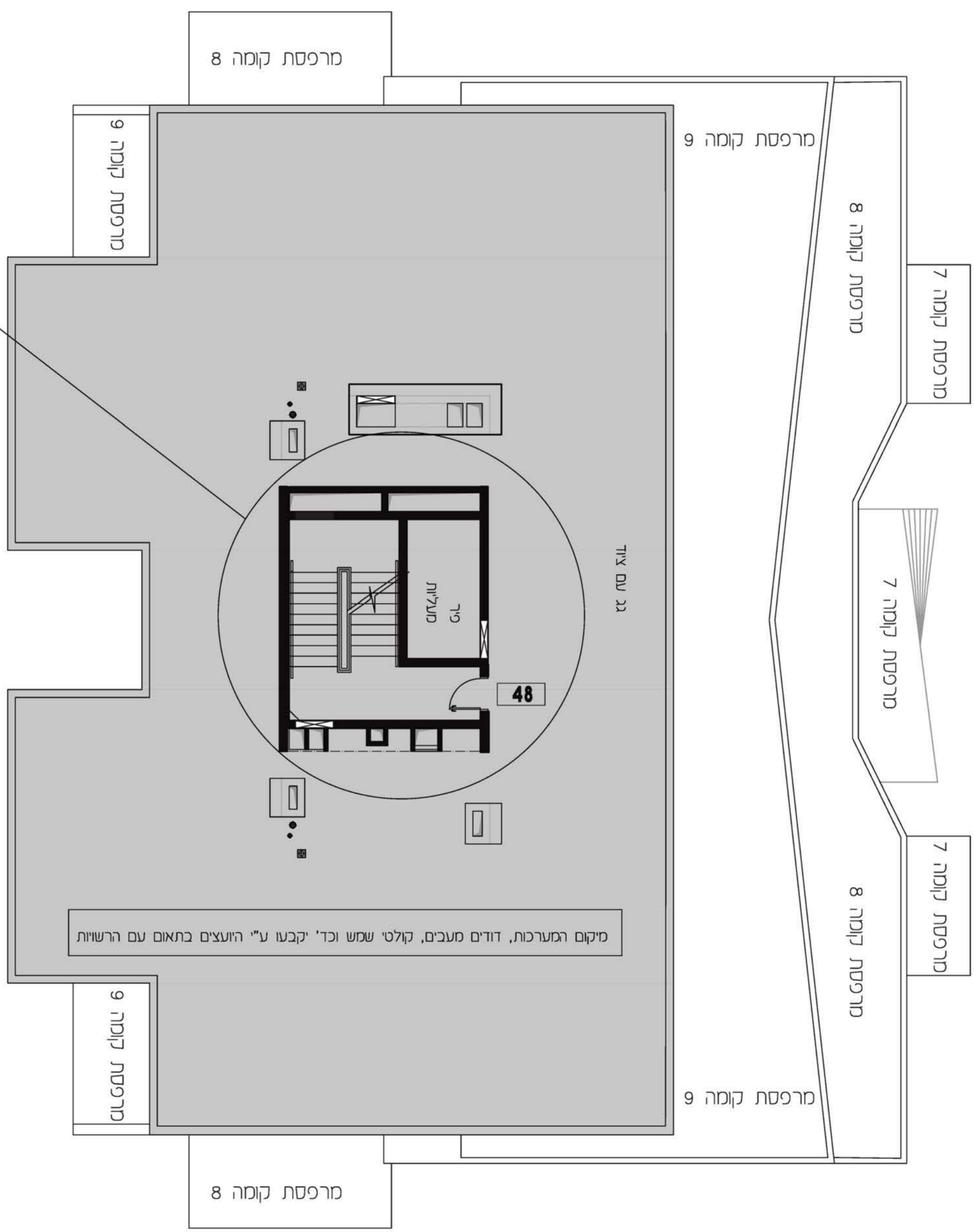
תכנית גג עליון
