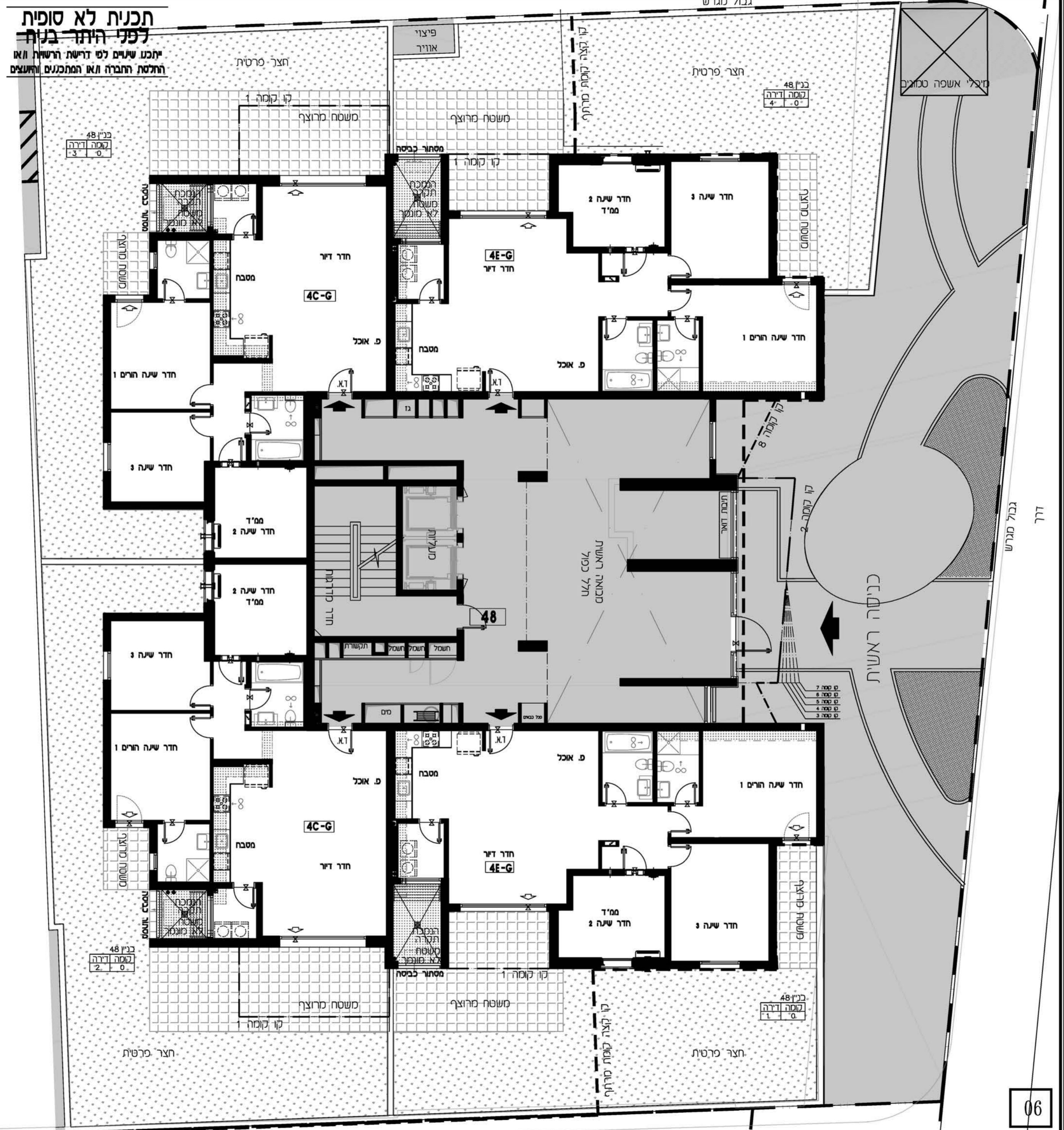
תכנית העמדה שכמטית מתחם ד
