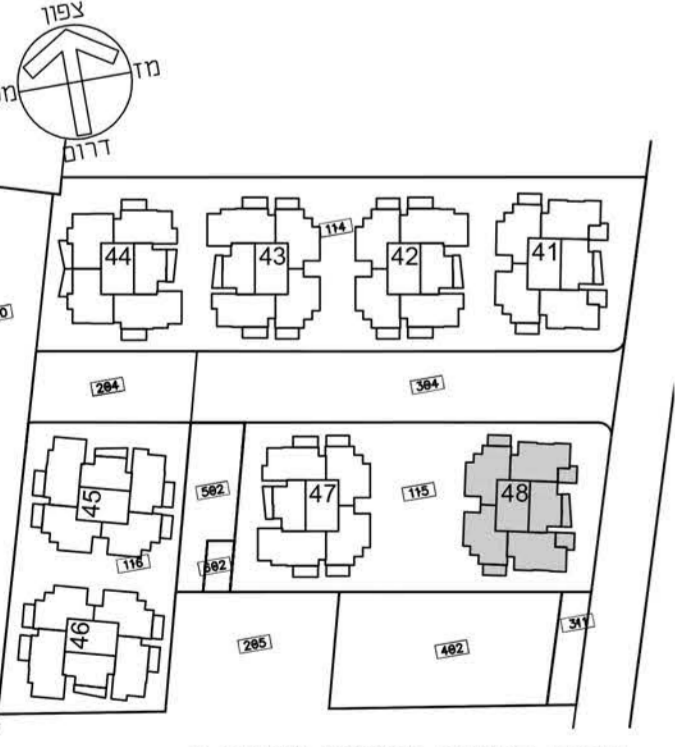
תכנית הגמדה סכמטית מתחם ד
