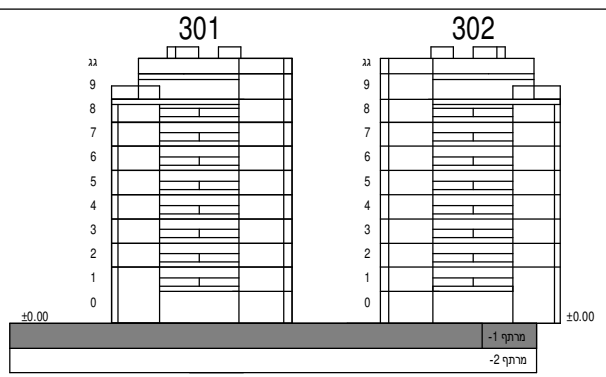
חתך סכמטי
