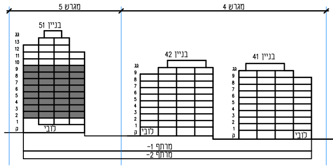
חתך סכמטי
