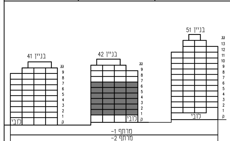
חתך סכמטי
