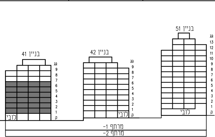
חתך טכני
