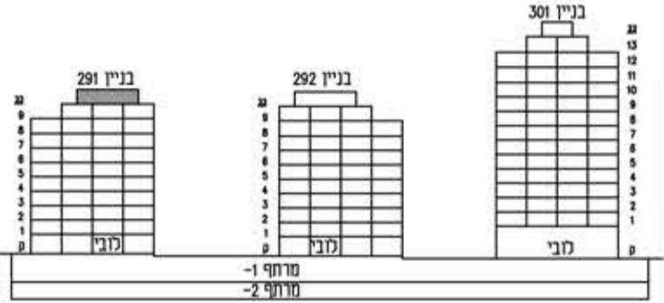
חזית סכמטית
