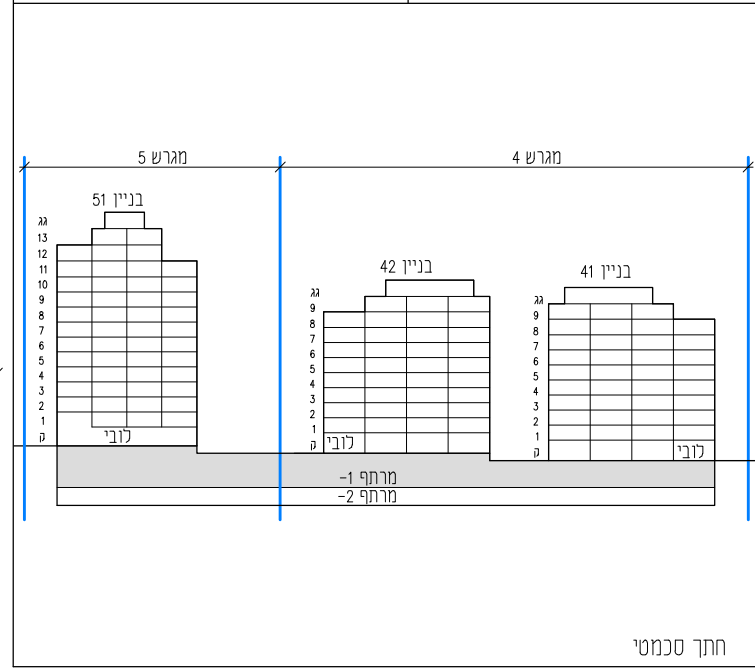
חתך סכמטי
