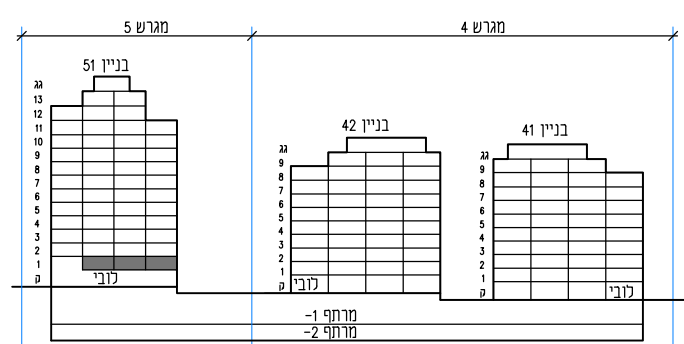
חתך סכמתי
