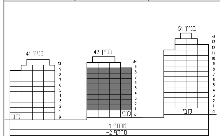
חתך סכמטי
