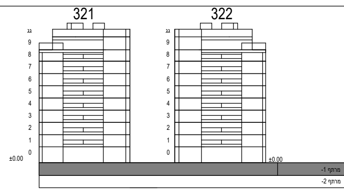
חותך סכמטי
