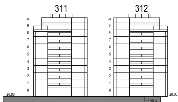
חתך סכמטי
