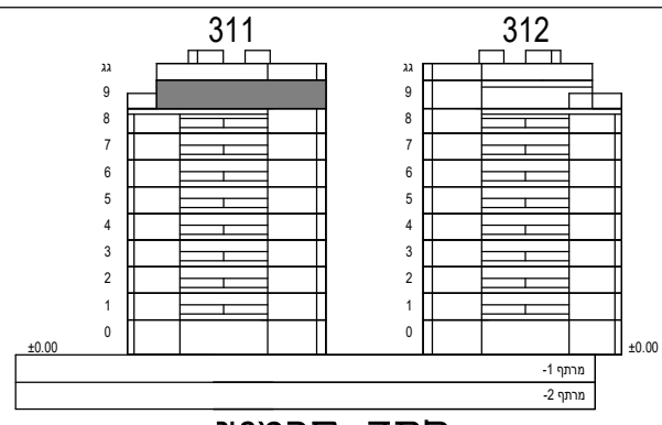
חותך סכמטי
