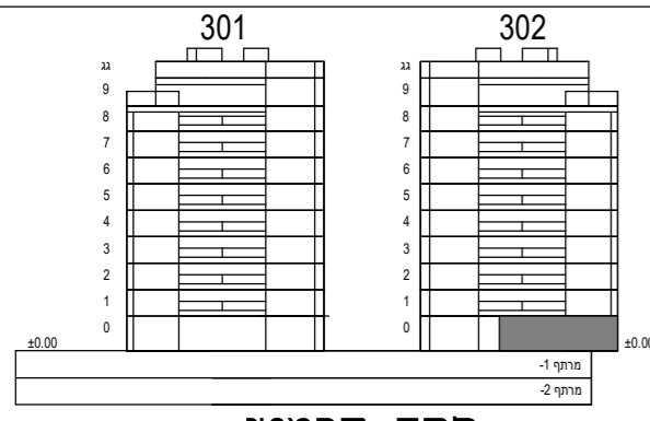
חתך סכמטי
