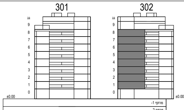
חתך סכמטי
