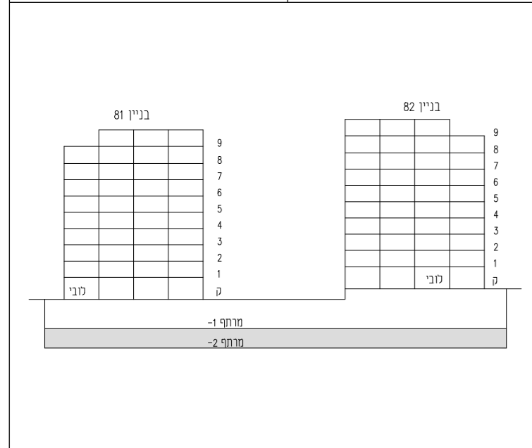
חתך טכני
