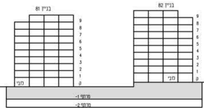
חזר סכמטי
